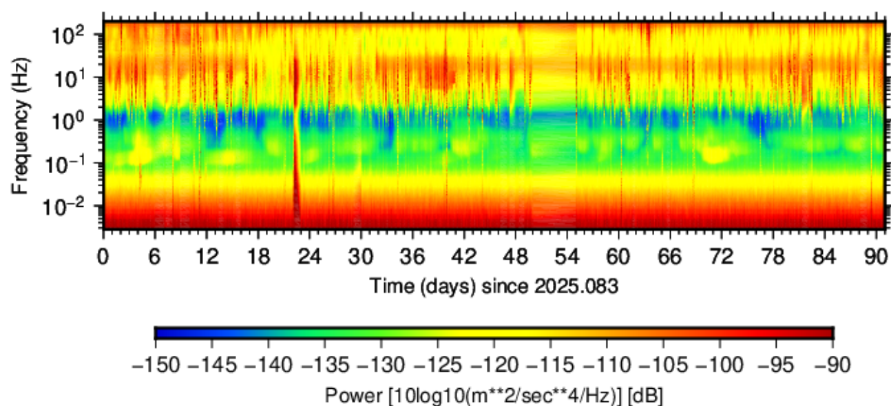
BG.AL4.DPE. (2025.083 - 2025.173)
