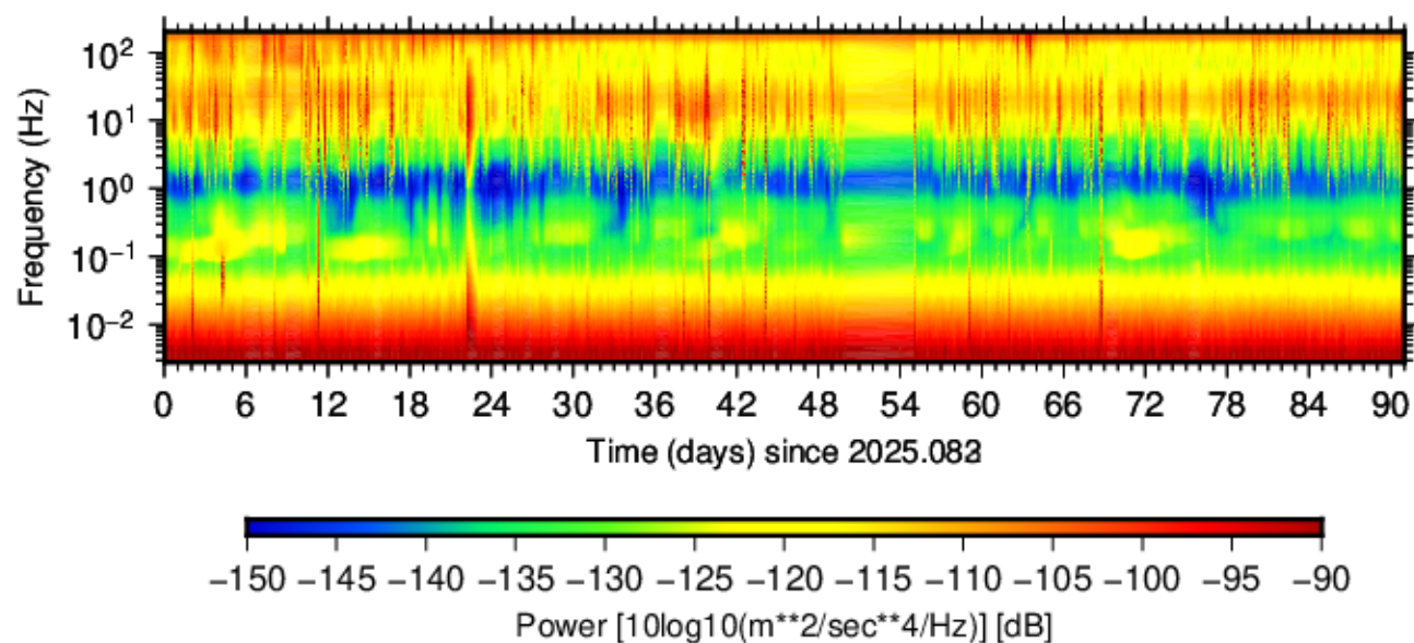
BG.AL4.DPZ. (2025.083 - 2025.173)
