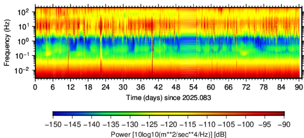
BG.AL4.DPN. (2025.083 - 2025.173)
