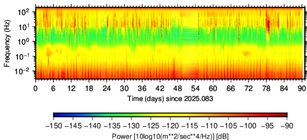
BG.ACR.CNE. (2025.083 - 2025.173)
