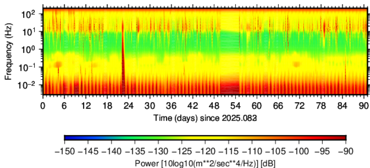
BG.ACR.CNZ. (2025.083 - 2025.173)
